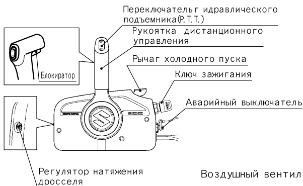
УЗЕЛ ДИСТАНЦИОННОГО УПРАВЛЕНИЯ
